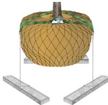
Baumverankerungssysteme: Deadman Plati-Mat & Spezial-Gurtband
